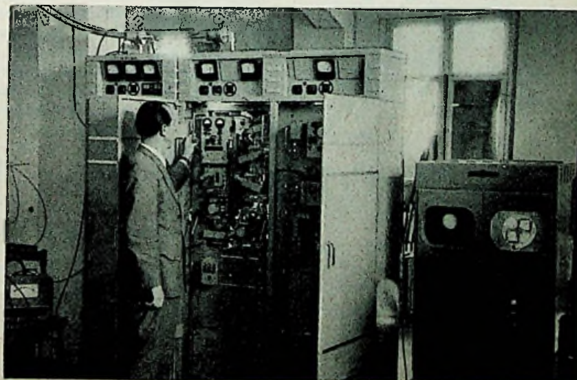
Telefunken-apparatuur in het eindstation Keulen
