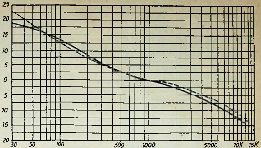
Fig. 1. De nieuwe standaardcurve met in vergelijking de als stippellijn weergegeven AES-curve.
